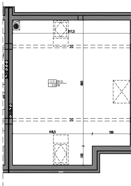
RZUT PODDASZA NIEUŻYTKOWEGO LOKAL L1
