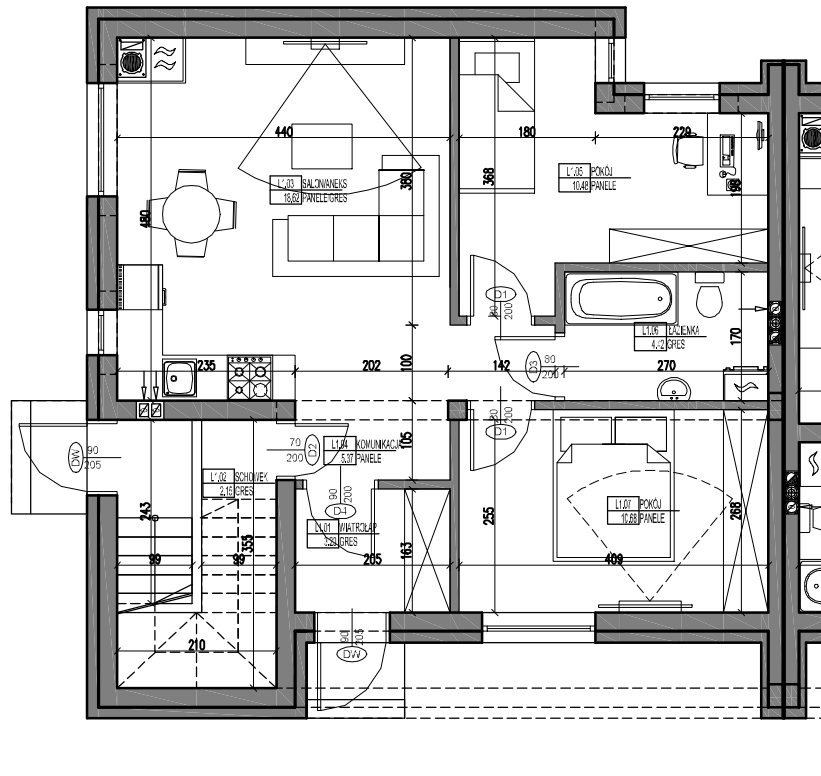
RZUT PARTERU LOKAL L1
