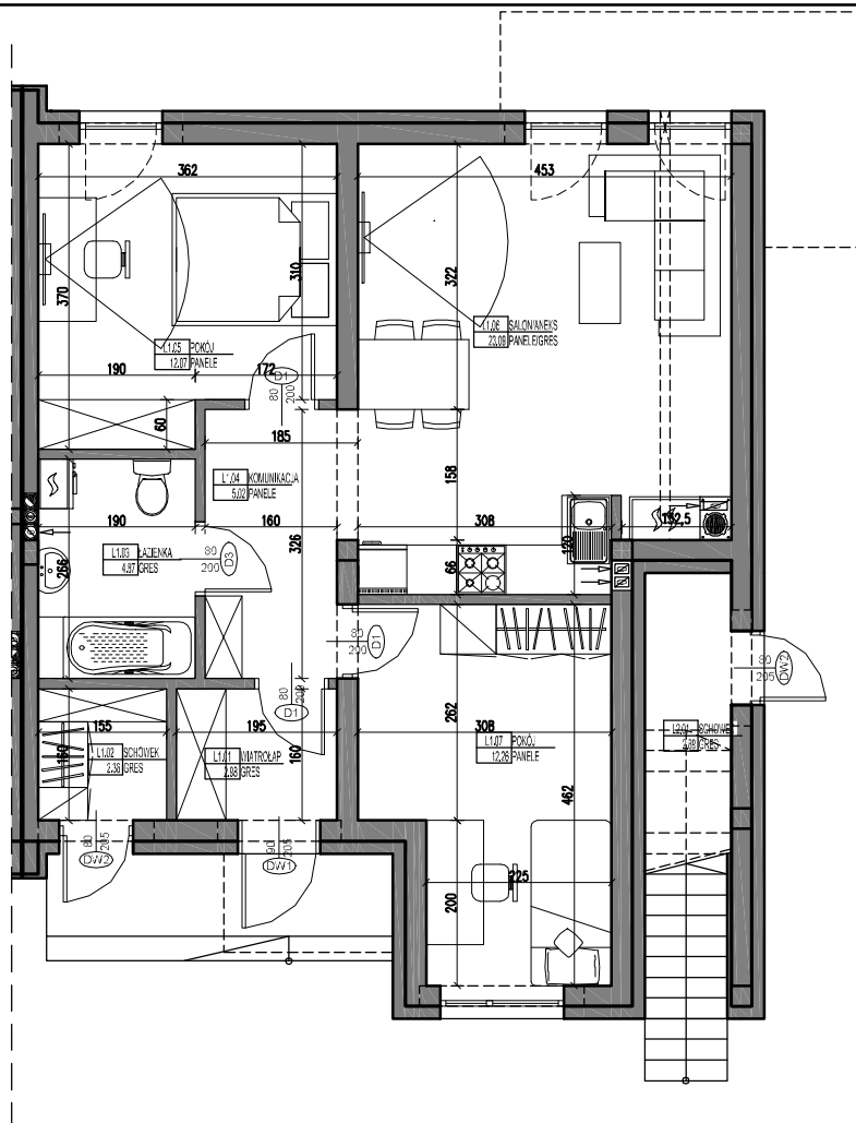
RZUT PARTERU LOKAL L1
