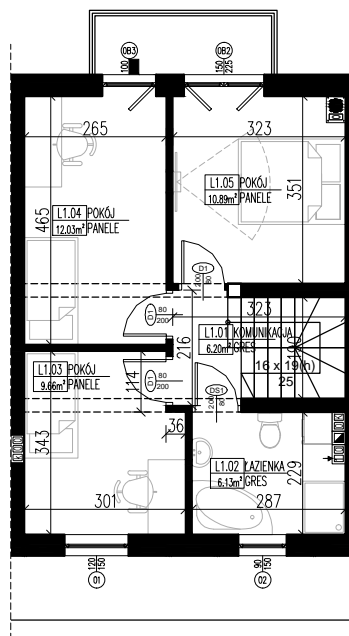
RZUT PIĘTRA
