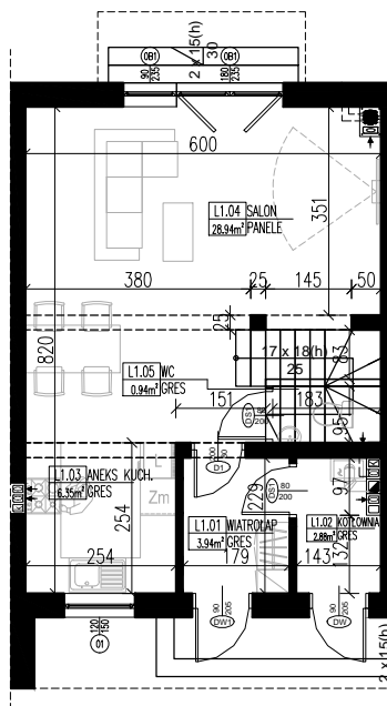
RZUT PARTERU
