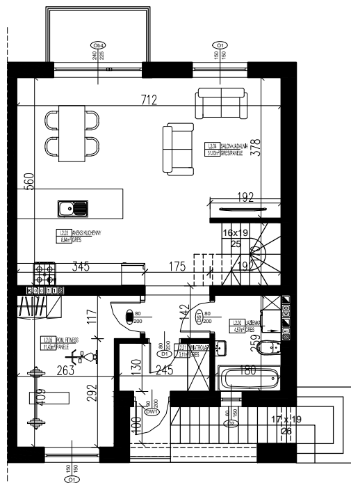
RZUT PIĘTRA
