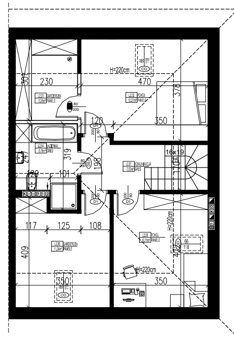
RZUT PODDASZA
