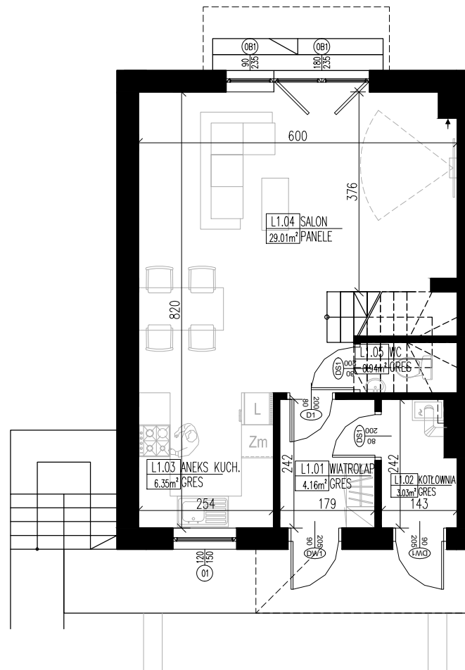
RZUT PARTERU
